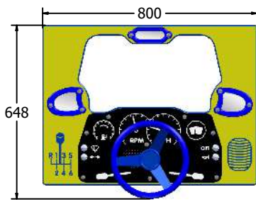
AMVFA-AP-FIPTDRIVE6-B
