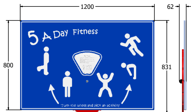
AMVFA-AP-FIACTWHEEL3
